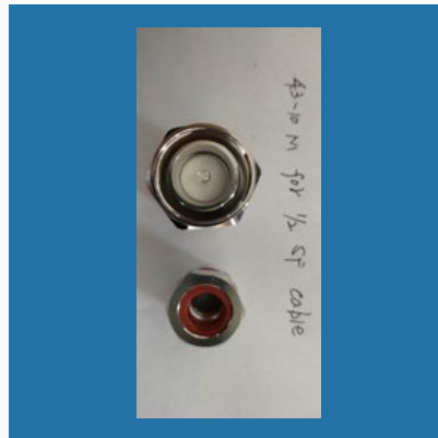
4.3/10 M For 1/2"SF Cable
